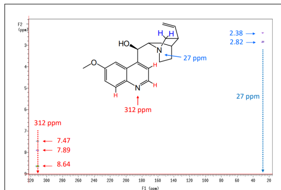
Figura 40: Spettro HMBC del chinino, riportato in figura con evidenziati color coded i segnali
