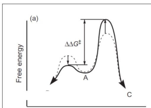
Figura 16: In tratteggiato, TS senza matched pair.
