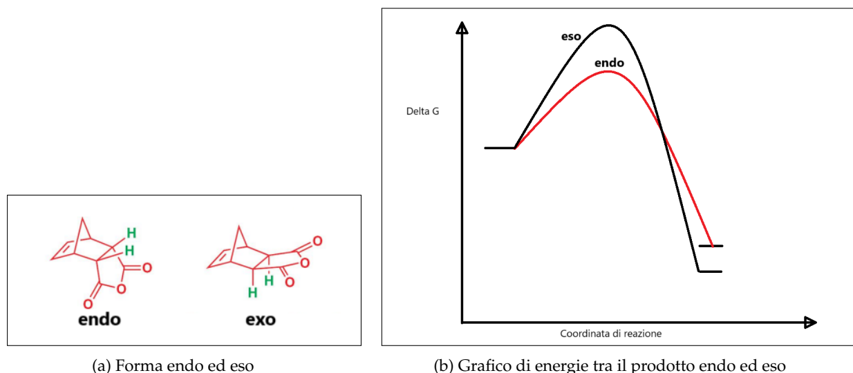
Figura 22: Confronto tra le forme endo/esso e il grafico di energie
