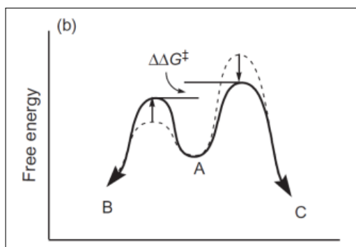
Figura 17: In tratteggiato, TS senza mismatched pair.
