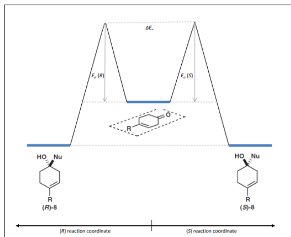
Figura 5: Stati di transizione enantiomerici.
