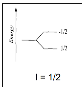
Figura 25: Stati possibili per un nucleo di spin \frac{1}{2} : \frac{1}{2} = \alpha , -\frac{1}{2} = \beta
